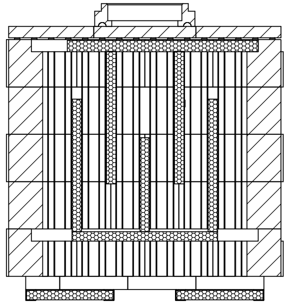
A-A (1 : 10)
