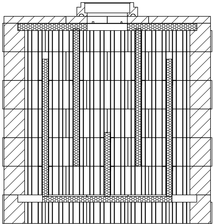
A-A (1 : 10)
